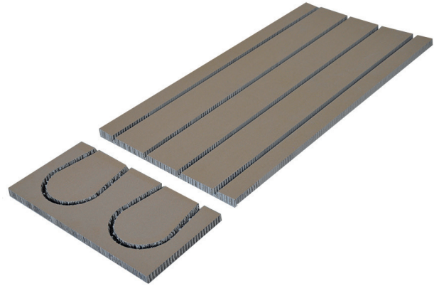
Rohrabstand 125 mm
